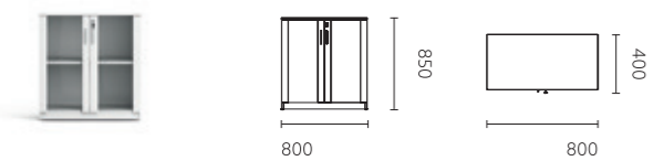
FKD30.08 800x400x850
